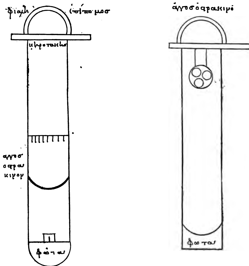
FIGURES 20 et 21. — Vases à digestion cylindriques. — Réda
